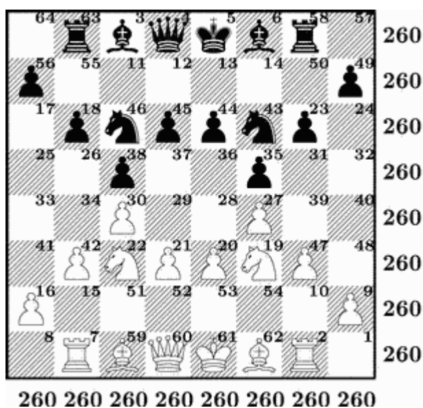
Рис. 1. Альмуджаннах и магический квадрат.
